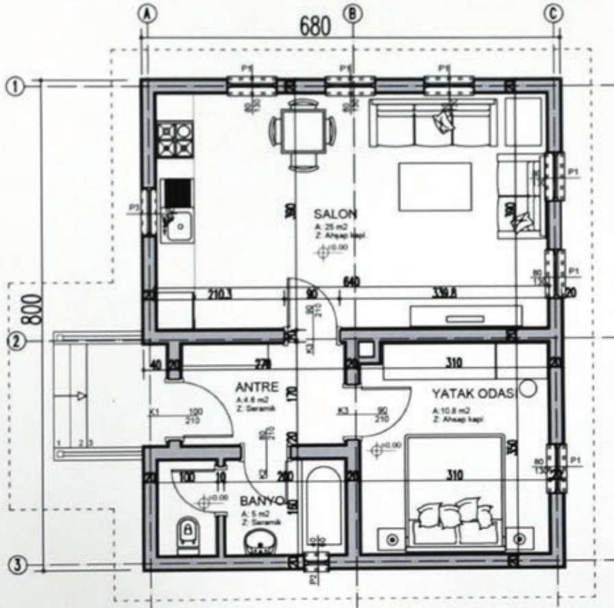
Zemin Kat Planı
