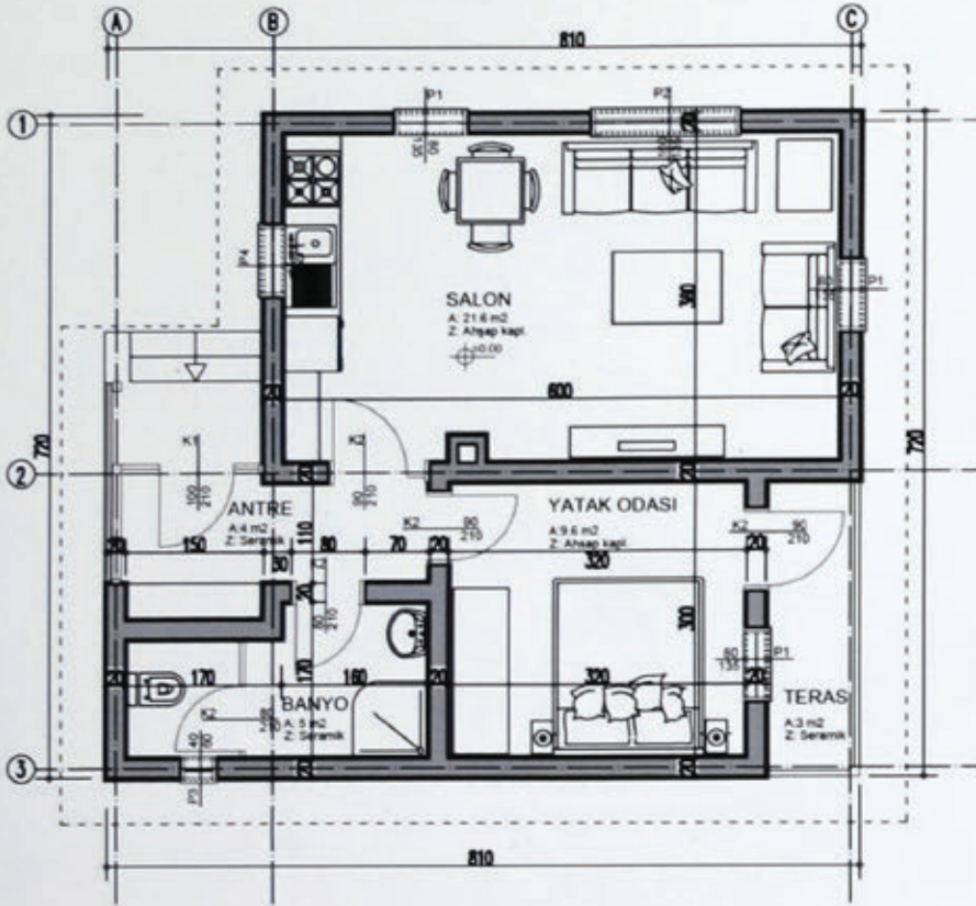
Zemin Kat Planı
